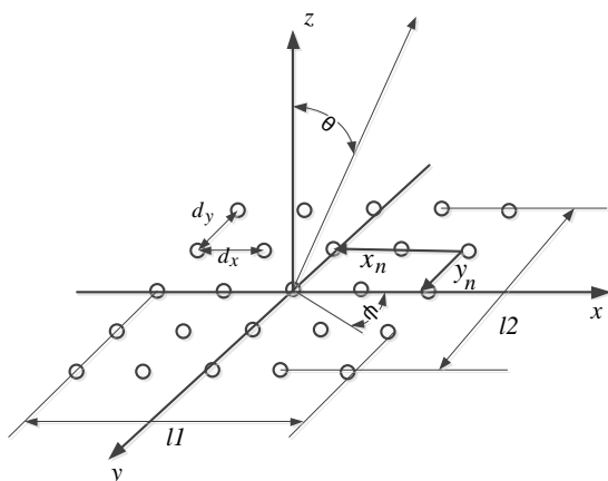
Рис. 2. Антенна решітка
