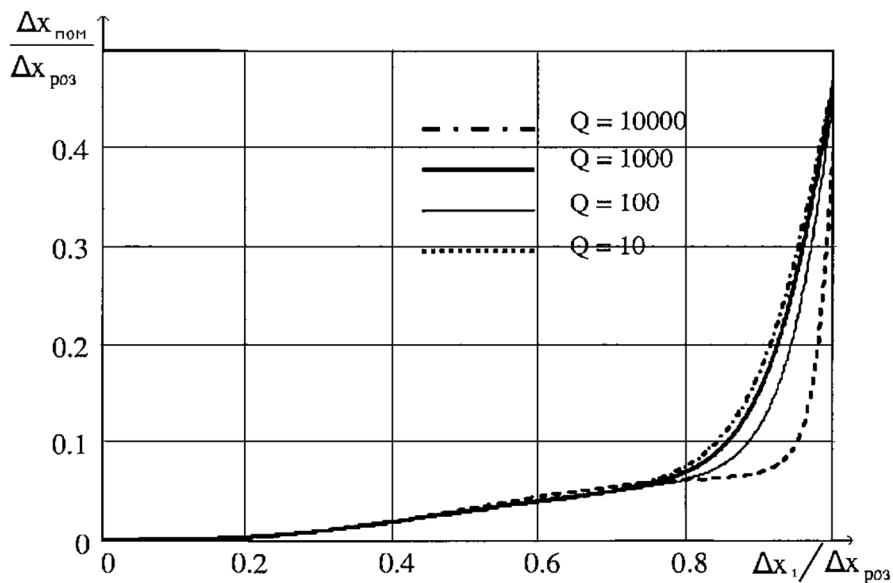
Рис. 2. Нормована залежність помилок похибки вимірювання від частоти, нормованої до інтервалу роздільної здатності, при використанні ВФ Дольфа-Чебишева
