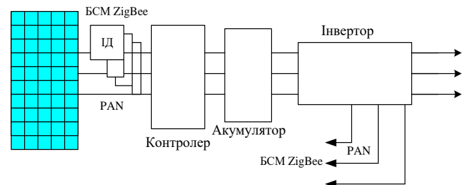
Рис. 2. Схема розподіленої САК ПФС
