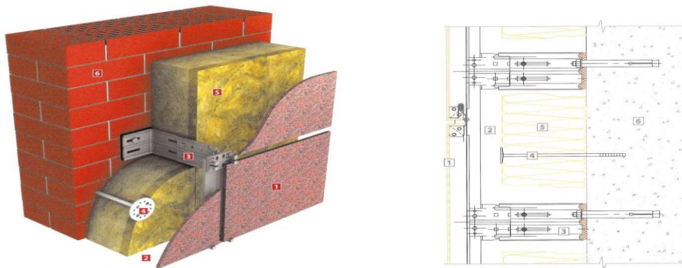
Рис. 2. Система вентильованого фасаду:
