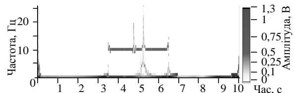
Гільберт-спектр сигналу s_1 .
