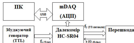
Структурна схема вимірювального каналу
