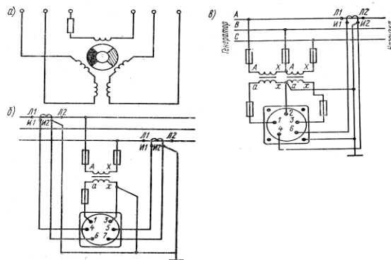
Принципова схема (а) і схеми включення електромагнітних фазометрів E 150 (б) і E160 (в).
