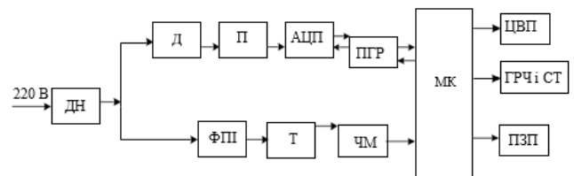
Структурна схема вимірювального каналу.
