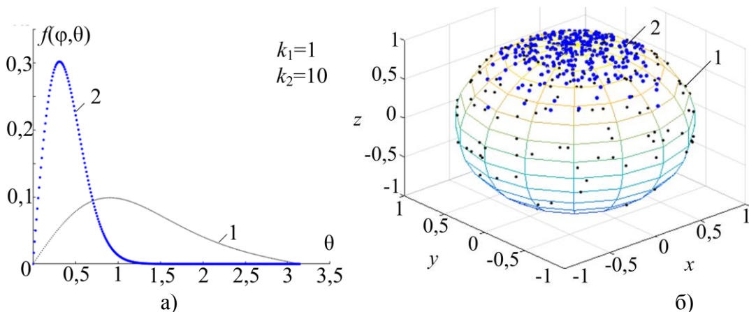
Рис. 1 – Розподіл Фішера на сфері: а) проекція функції розподілу ймовірностей на вісь \theta ; б) вибірки випадкових векторів
