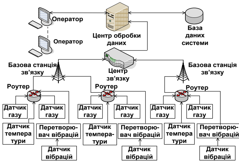
Рис. 1 – Структура телекомунікаційної системи моніторингу магістральних газопроводів
