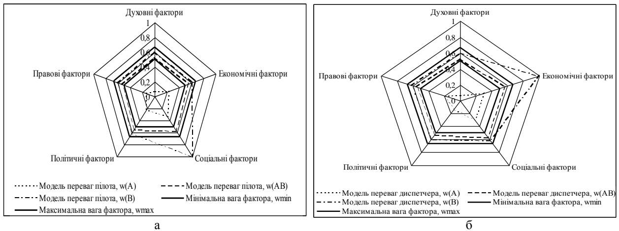
Рис. 5. Моделі переваг пілотів (а) і диспетчерів (б) ЦА у разі вибору у бік позитивного полюсу w(A) , негативного полюсу w(B) та однакового тиску при виборі в бік позитивного і негативного полюсів w(A)=w(B)=w(AB)
