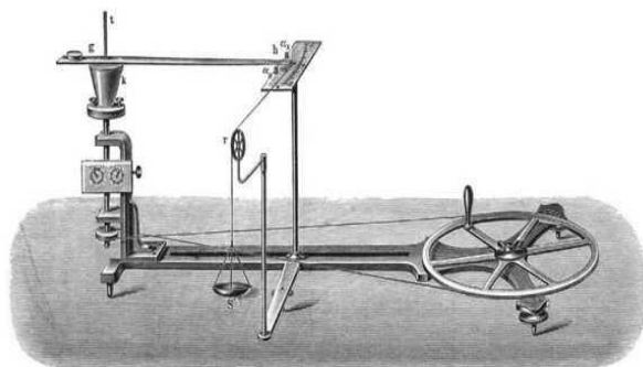
Рис. 10.8. Прилад Пулюя для досліджень
