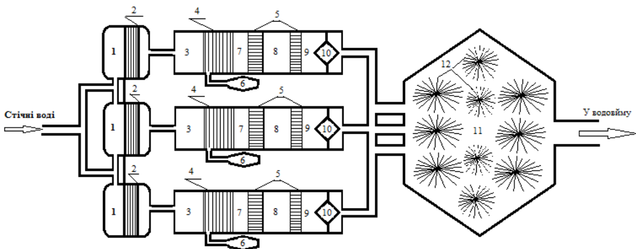
Рис. 3. Модернізована технологічної схеми очищення виробничих стічних вод:
