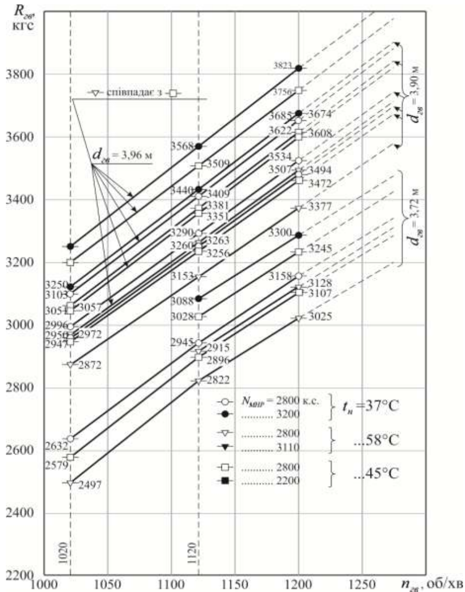
Рисунок 4.14 – Залежність тяги від обертів повітряного гвинта. Максимальний надзвичайний режим: R_{в\ мнр} = f(N_{в\ мнр}, t_n^0, n_{в}, d_{в}) при N = 0, M_{п} = 0 . Джерело: дані ВАТ НВП «Аеросила»
