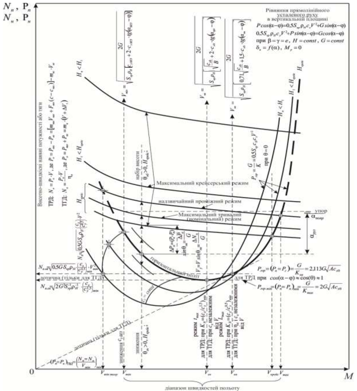
Рисунок 4.3 – Схема використання методу потрібних і наявних тяг у моделях узгодження змін у крилі й силевій установці
