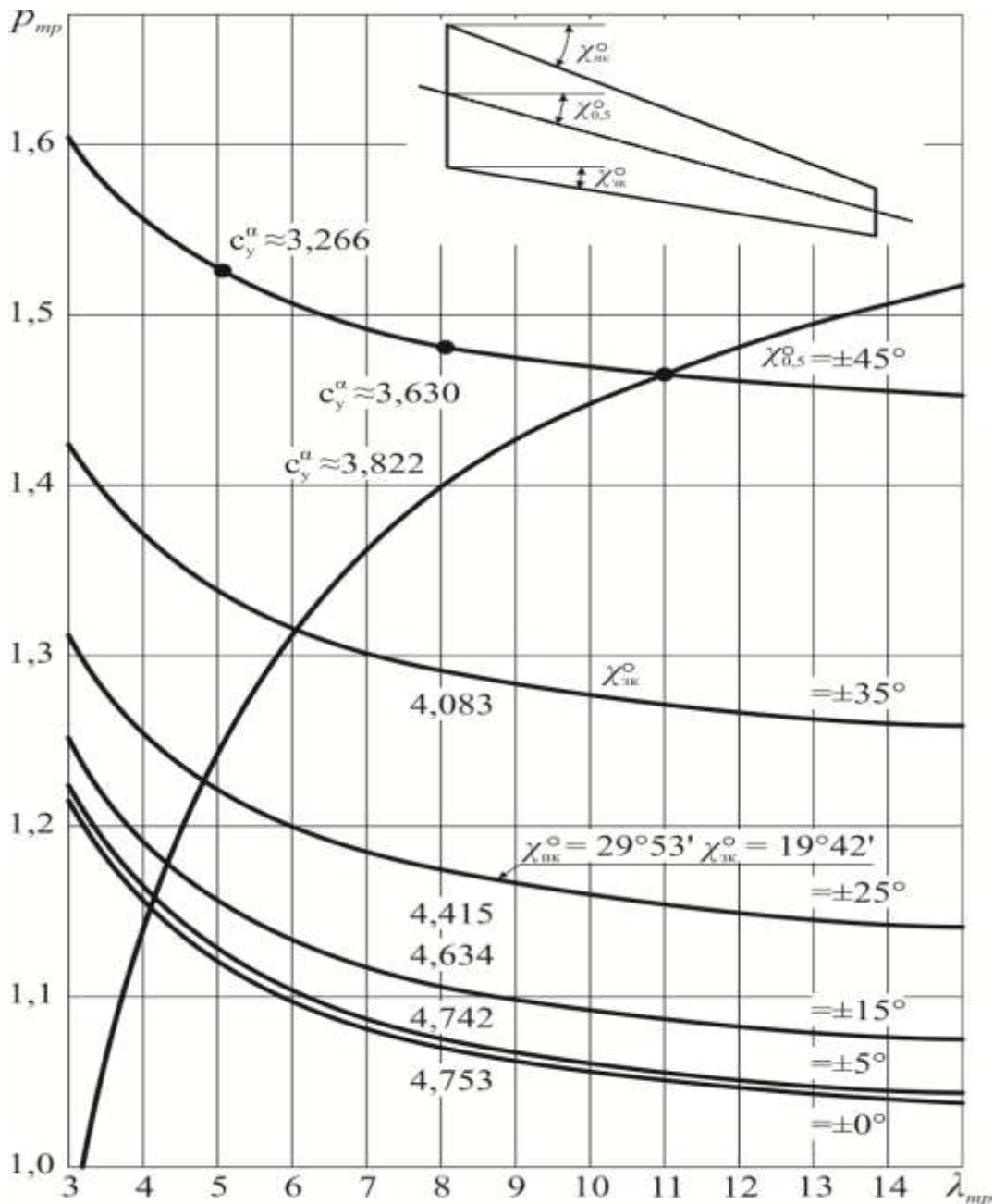
Рисунок 2.5 – Вплив зміни геометричних параметрів на несну здатність стрілоподібного крила C_y^\alpha при \eta_{tr\text{opt}} \approx 2,899
