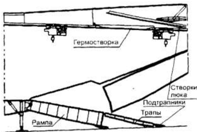
Вантажний люк у відкритому положенні на землі
