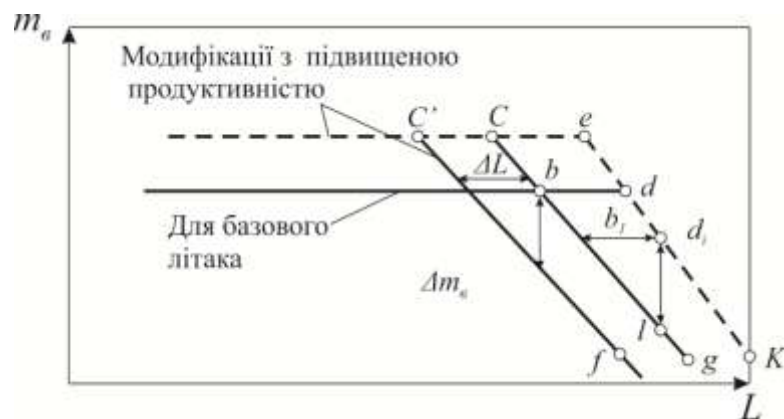
Рисунок 1.3 – Зміна характеристик «вантаж – дальність» при розробці модифікацій базового літака
