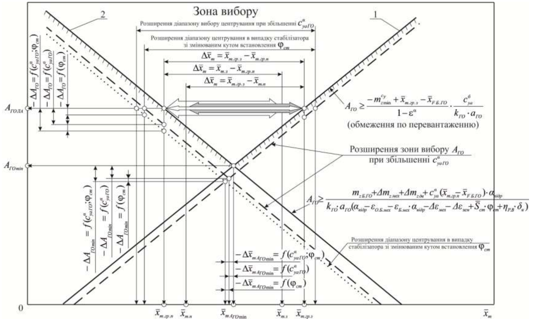
Рисунок 3.12 – Граничні лінії та область вибору параметрів A_{ГО} і \bar{x} : 1 – мінімально допустимий ступінь поздовжньої статичної стійкості; 2 – балансування літака на великих кутах атаки крила [84]
