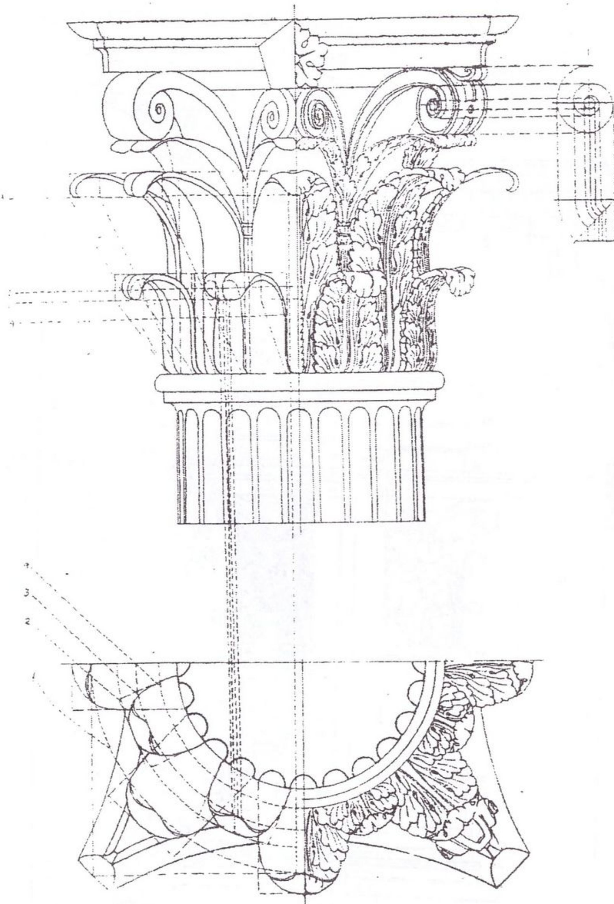
Рис. 10. Деталі коринфського ордеру
