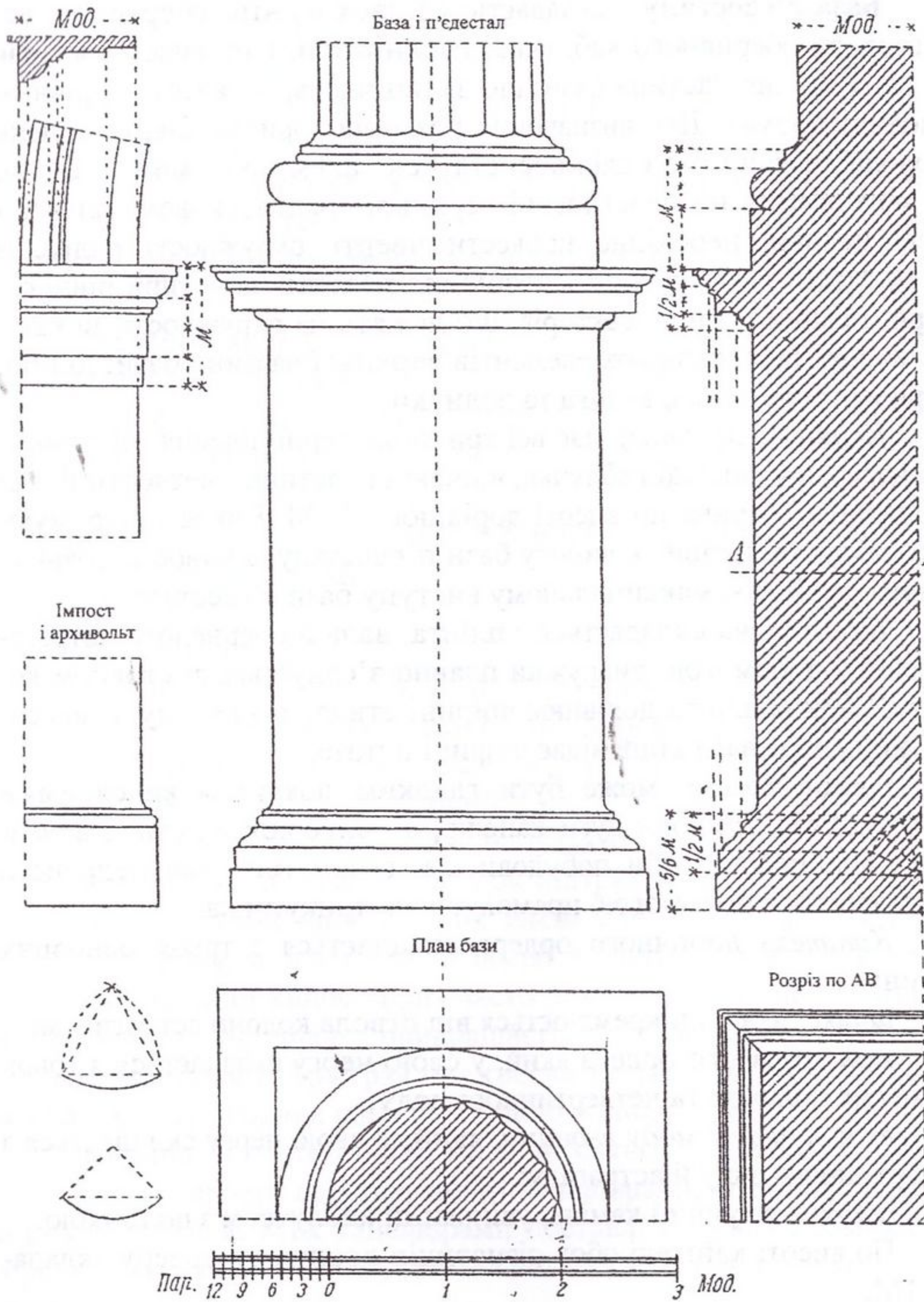
Рис. 8. Деталі доричного ордеру
