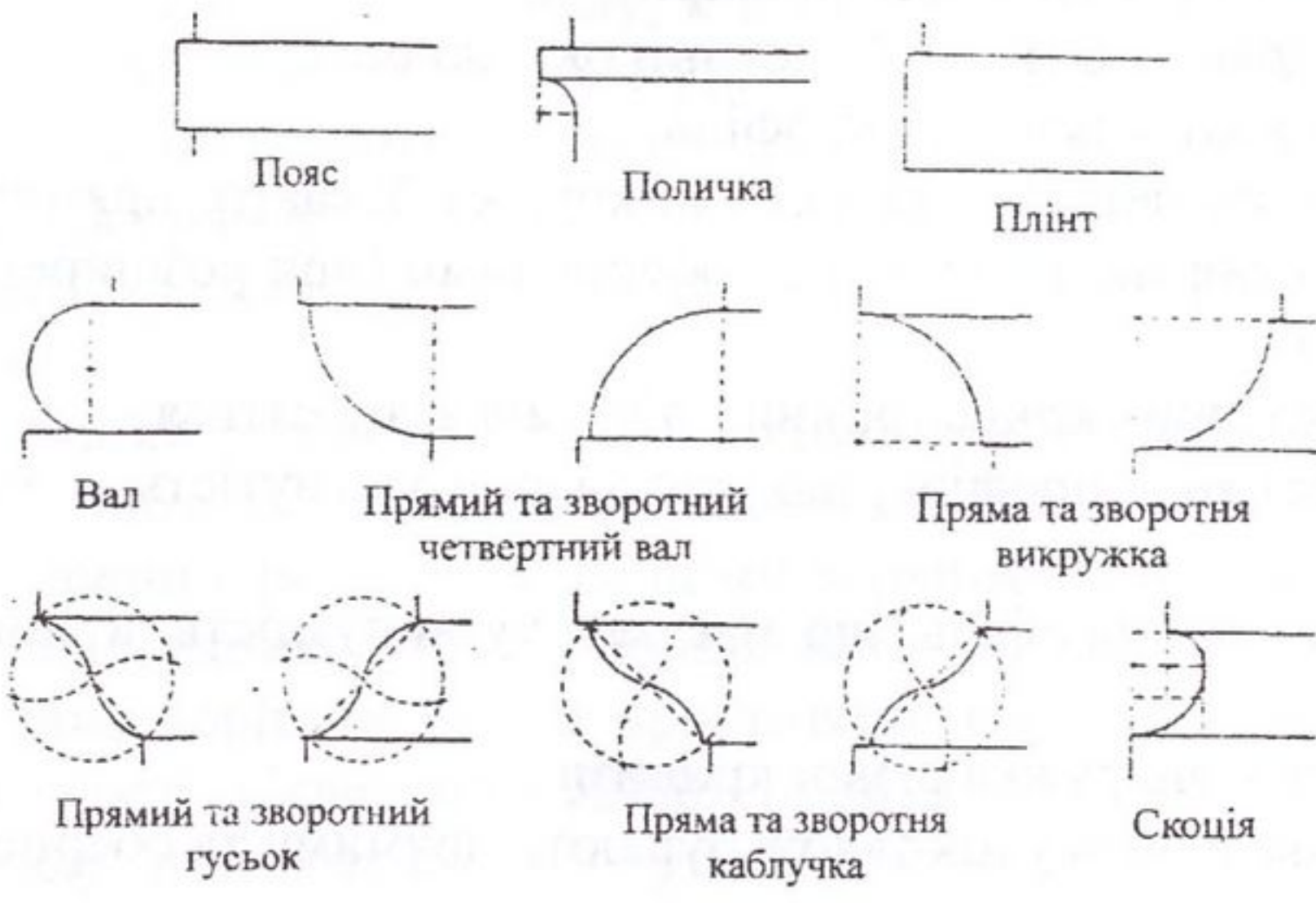
Рис. 6. Прямолінійні та криволінійні обломи
