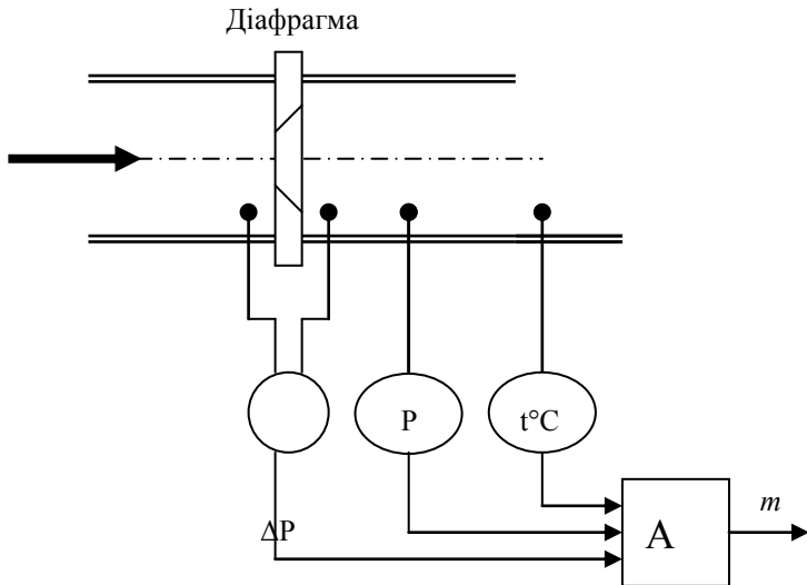
Рис. 12. Приклад компенсації мультиплікативних завад (тиску і температури) при вимірюванні витрати за допомогою вимірювальної діафрагми; A – керуючий обчислювач.
