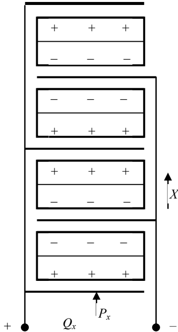
Рис.20. Чутливий елемент з декількома кварцовими пластинами
