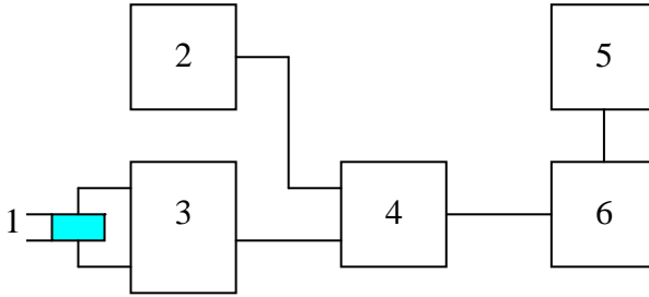
Рис. 31. Вимірювання температури за допомогою кварцового генератора частоти.
