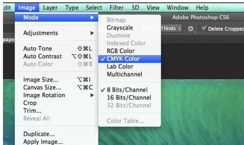
Рис.2.3. Колірний режим
