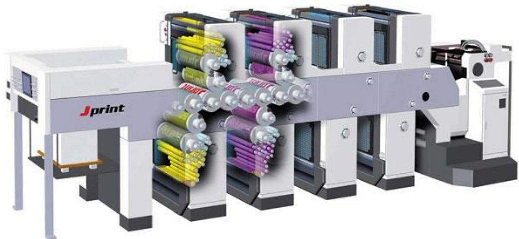
Рис.1.13. Будова сучасної офсетної машини [22]
