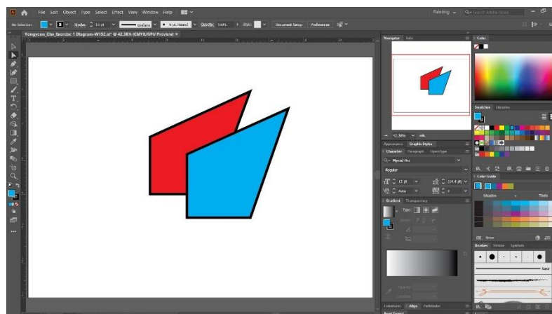
Рис.2.6. Інтерфейс Illustrator
