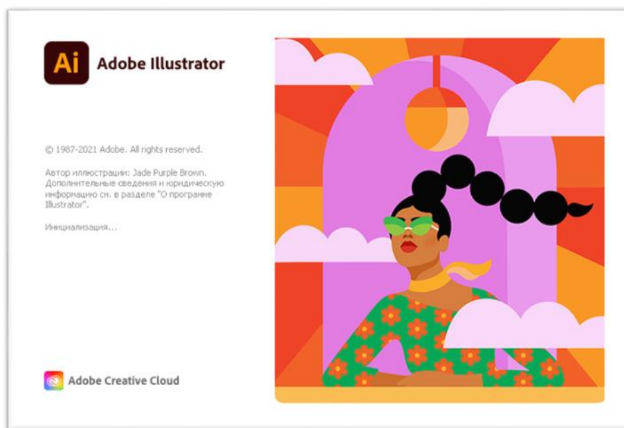
Рис.2.5. Adobe Illustrator
