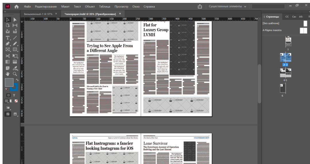
Рис.2.1. Інтерфейс InDesign
