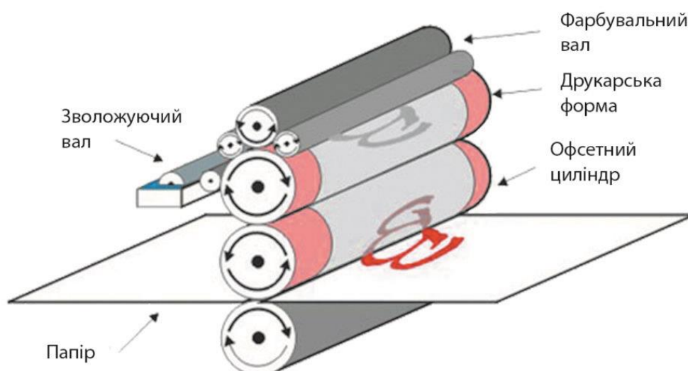
Рис.1.12. Схема принципу роботи офсетного друку [21]
